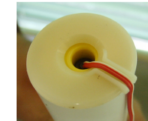
着火具を取り付けた状態、脚線ガイドの谷間に脚線をセットする
